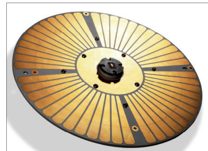
MEMSコンタクト技術によるDCパラメトリック測定用 Micro Spring Type "Takumi Pico™" (米国フォームファクター社製)
